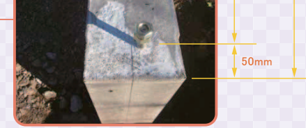
アンカーは基礎芯ではありません
